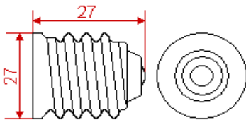
E27 Sockel-Layout E27 base layout
